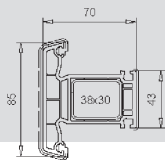
Setzpfosten 85mm 102.218 Stahl 113.271
