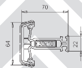
Flügelprofile 64mm 102.237 Stahl 113.020
