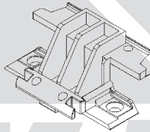
Pfostenverbinder M.1:2
