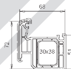
Aufbauprofil 72mm 103.208 Stahl 113.271
