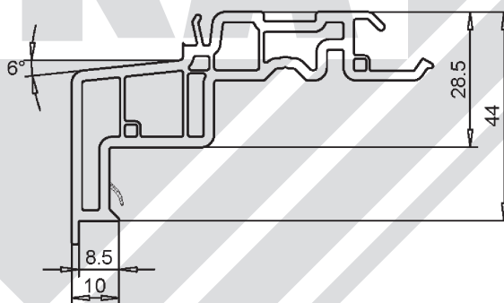
Kopplung waagrecht 116.212
