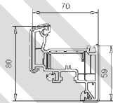
Flügel 80mm nitr. 103.277 Stahl 113.290 (weiss) Stahl 113.290.3 (farbig)
