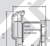
Flügel 118mm nitr. 103.283 Stahl 113.304
