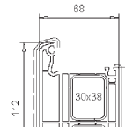
Aufbauprofil 112mm 105.201 Stahl 113.271
