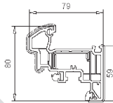
Flügel 80mm nitr. 103.278 Stahl 113.290 (weiss) Stahl 113.290.3 (farbig)
