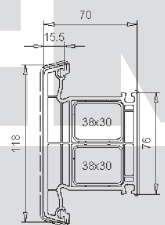
Setzpfosten 118mm 102.238 Stahl 113.271
