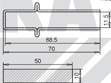
vorhandener VEKA Artikel 113.013.3
