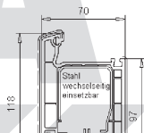
Flügel 118mm nitr. 103.279 Stahl 113.304
