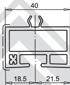
Aufbauprofil Art.-Nr. 108.008 für Art.-Nr.108.035.2 / 086
