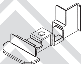
Endstück einteilig 109.519
