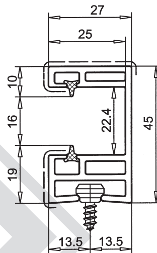
Rolladenführung
