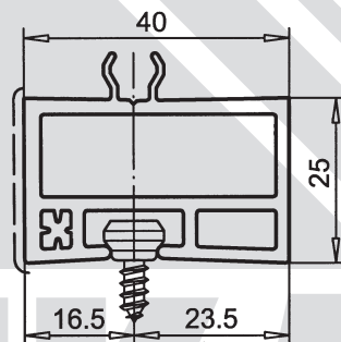
Aufbauprofil Art.-Nr. 108.008 für Art.-Nr. 108.005 / 014 / 062.2
