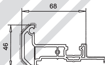
Losser Setzpfosten 46mm (für Falzhebel) 102.219
