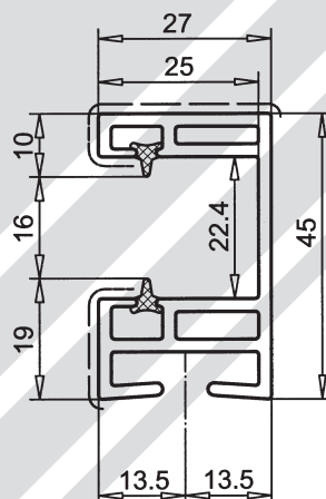
Aufbauprofil Art.-Nr. 108.087 für Art.-Nr.108.035.2 / 086
