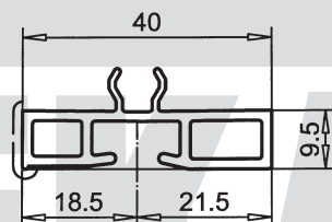
Aufbauprofil Art.-Nr. 108.087 für Art.-Nr.108.035.2 / 086
