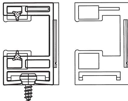
Einlauftrichter 108.033
