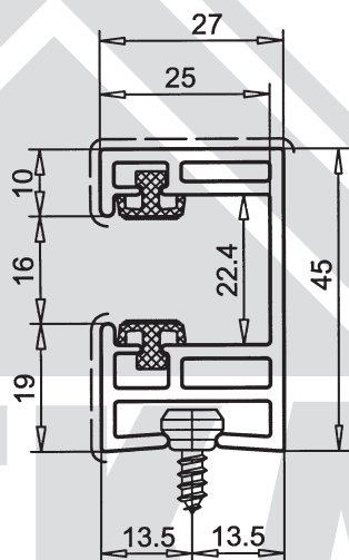
Rolladenführung
