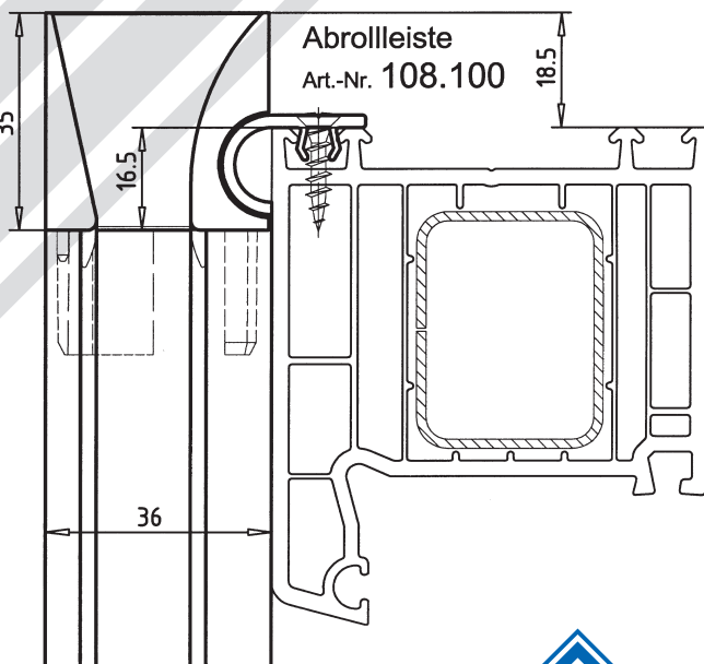
Einlauftrichter ausgenommen Art.-Nr. 108.103 / 108.104
