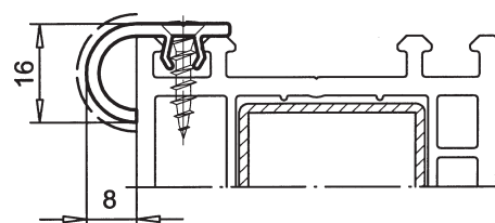
Abrollleiste Art.-Nr. 108.100
