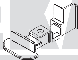
Endstück einteilig 109.509
