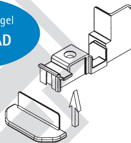
Endstück zweiteilig Innenteil 109.507.4
