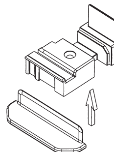
Endstück zweiteilig Innenteil 109.508.3 Farbe: weiss Aussenteil 109.508.2 Farben: braun, ockerbraun, schwarz, silbergrau, tannengrün
