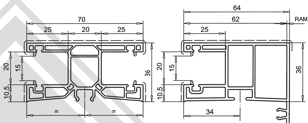
Doppelte Rollladenführung für Ausführung weiss:
