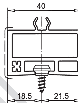
Aufbauprofil Art.-Nr. 108.008 für Art.-Nr. 108.035.2
