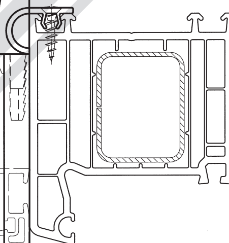
Abrollleiste Art.-Nr. 108.100
