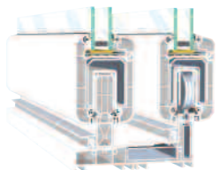
Profilé pour porte levante coulissante VEKA TOPLINE – stabilité et fonctionnement sans faille durant de longues années
