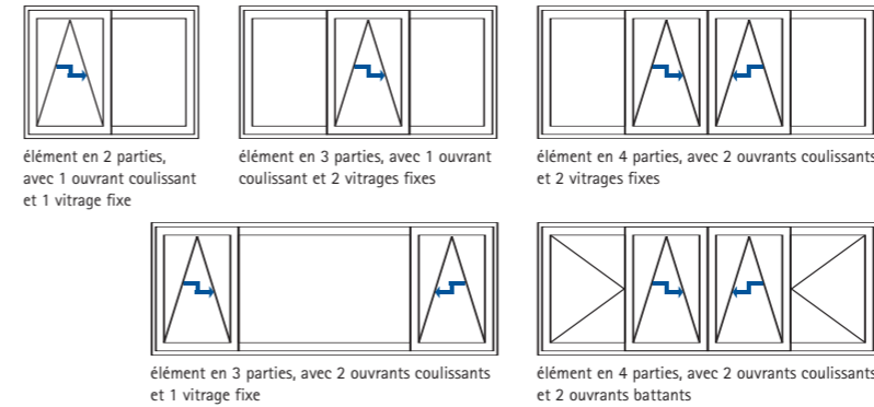
Variantes de la porte coulissante en translation
